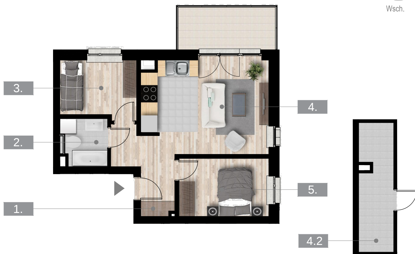
KOMÓRKA LOKATORSKA
